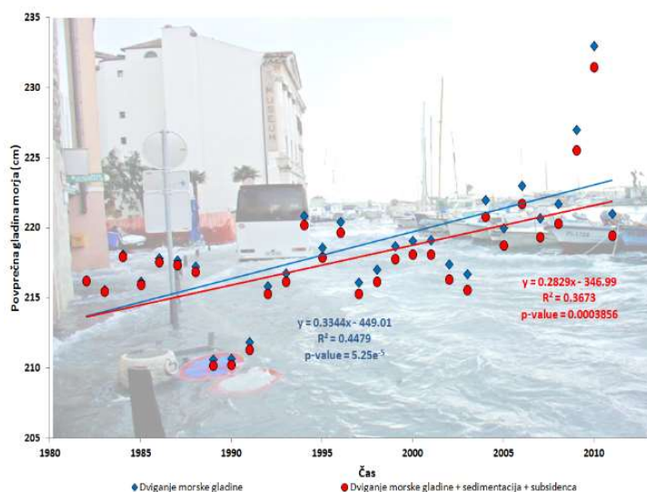
Figura 13: Innalzamento del livello del mare dal 1982 al 2011 (0,33 cm/anno; linea blu) a Capodistria (ARSO, 2011) e tendenza aggiustata (a) con sedimentazione (0,053 cm/anno) e subsidenza (0,0015 cm/anno) e previsioni di innalzamento del livello del mare secondo il Quinto rapporto IPCC (b)
