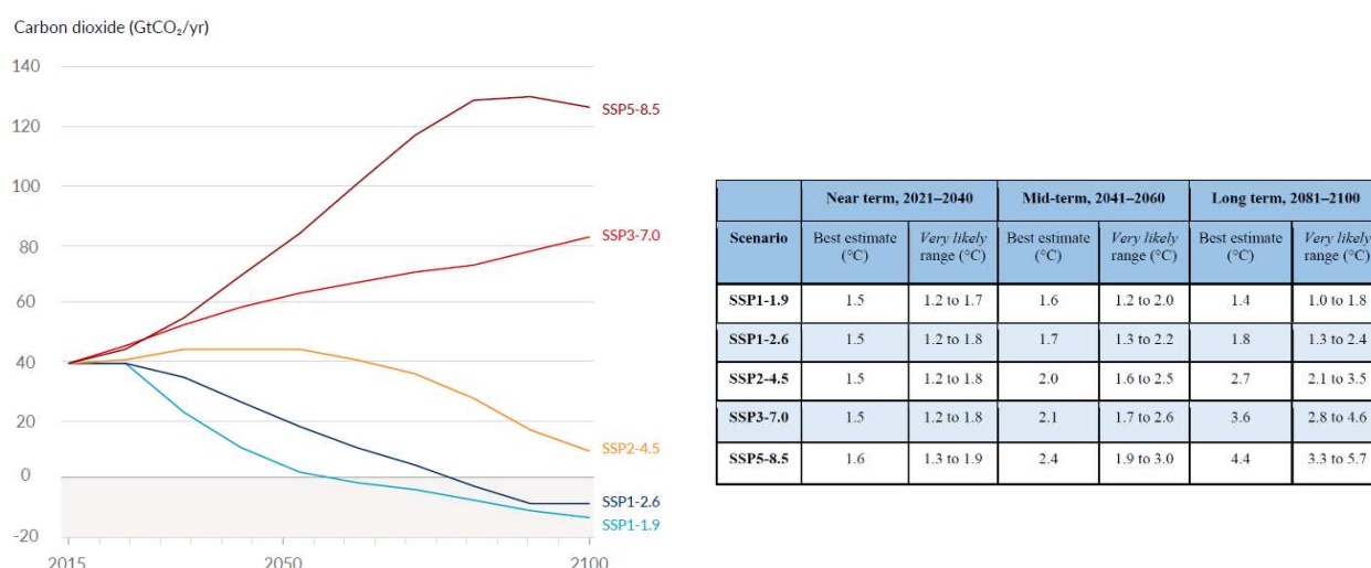
Figura 2: Le emissioni annuali di CO 2 in futuro, secondo i cinque diversi scenari (a sinistra) e le variazioni della temperatura superficiale globale in periodi ventennali selezionati sulla base dei cinque scenari di emissione considerati (a destra) (IPCC 2021)
