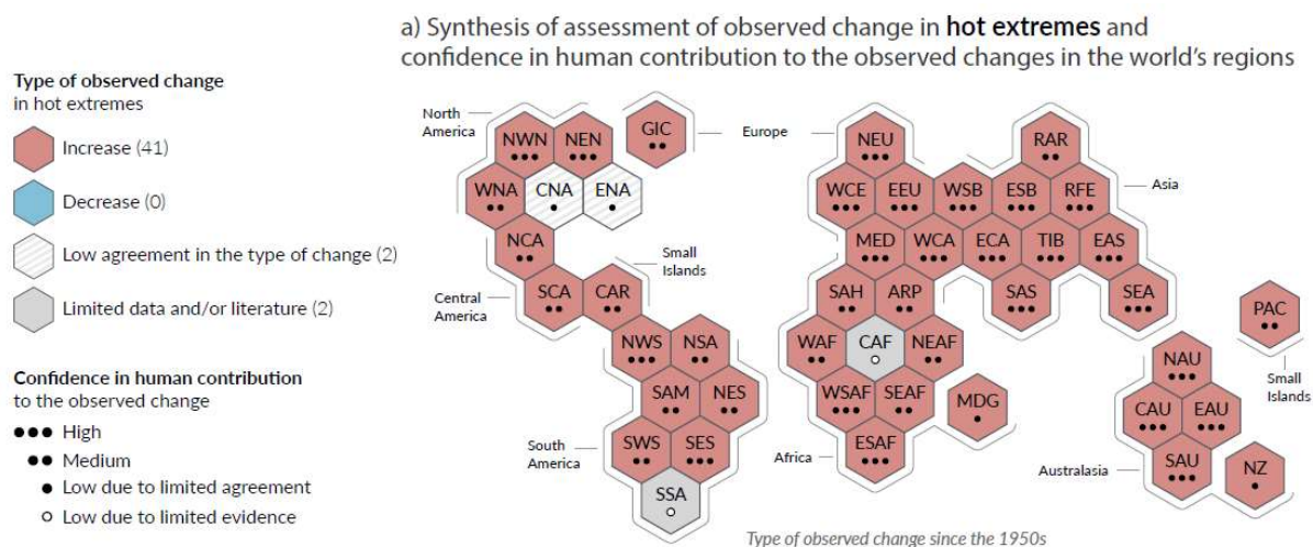
Figura 3: Stima dei cambiamenti osservati nelle temperature estreme per regione, mostrata secondo la categorizzazione IPCC AR6 WGI (IPCC 2021)
