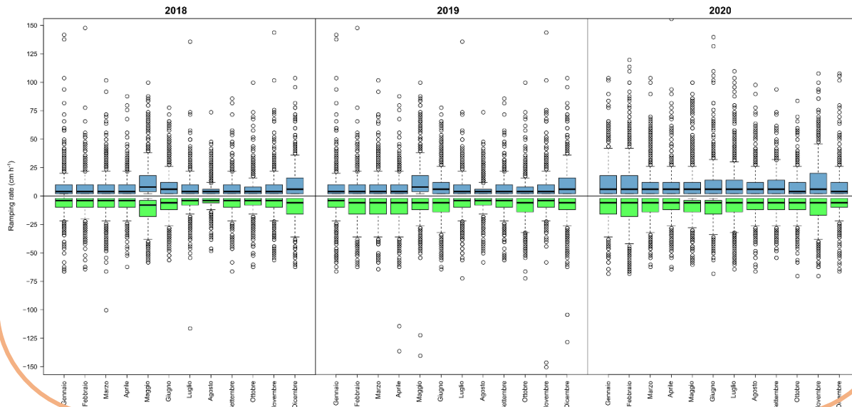
Porazdelitev „Ramping Rate“ vrednosti ( \text{cm h}^{-1} ) Gorica hidrometer (2018 - 2020)
