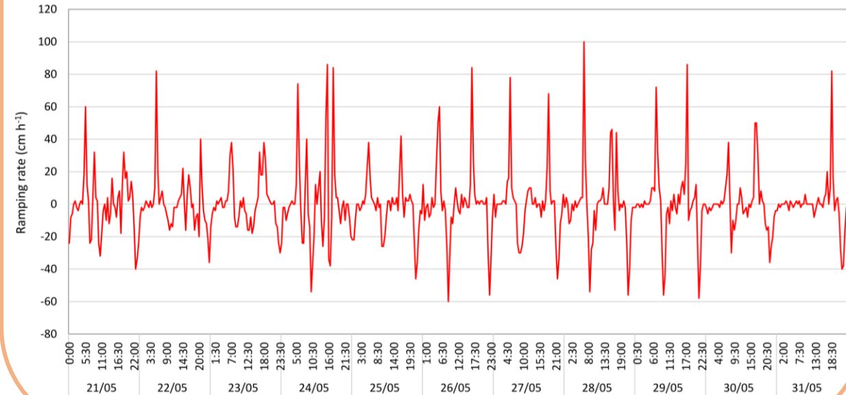
Vrednosti „Ramping Rate“ ( \text{cm h}^{-1} ) Gorica hidrometer (Maj, 21-31, 2020)
